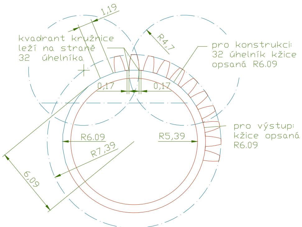
DETAIL KONSTRUKCE OZUBENÉHO KOLA
