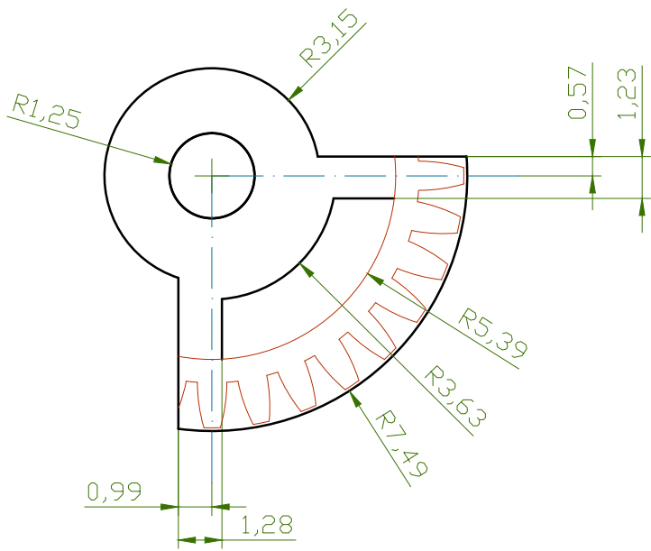
DETAIL STŘEDOVÉ ČÁSTI
